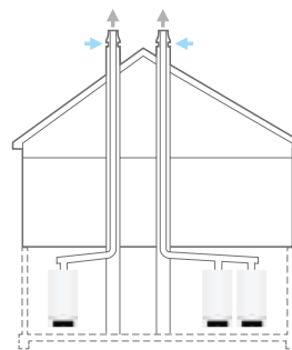
Beispiel Alt- oder Neubau, bei dem ein vorhandener Schornstein oder Schacht zur Luftansaugung geeignet ist. Links raumluftunabhängig mit eingezogenem Abgasrohr im Kamin, rechts bei vorhandenem Abgasschacht im Kamin (Einfachbelegung).
