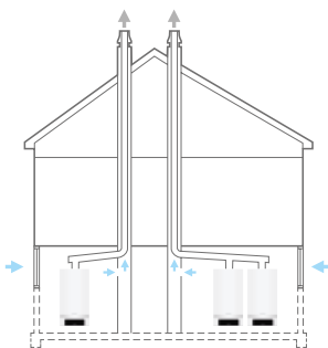
Beispiel Altbau, bei dem ein vorhandener Schornstein oder Schacht nicht zur Luftansaugung geeignet ist. Raumluftabhängige Einfachbelegung (links) bzw. Kaskade (rechts).
