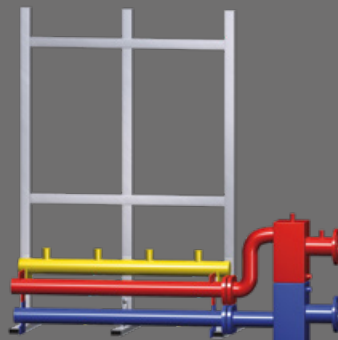
2. Schritt: Einzelteile der Anschlussgruppe einfach installieren.
