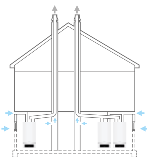
Beispiel Altbau, mit vorhandenem, aber kleinerem Schacht oder Schornstein. Abgasabführung unter Überdruck, raumluftunabhängiger Betrieb über Luftansaugung mit separatem Zuluftrohr. Überdruckkaskade mit Abgasklappe zur Reduzierung der Abgasdurchmesser.
