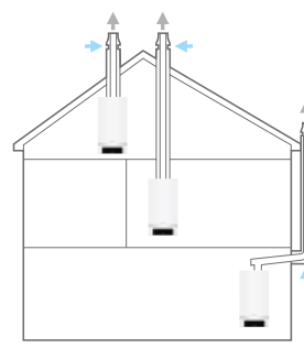
Einsatzbereich Neu- oder Altbau ohne vorhandenen Schornstein oder Schacht. Raumluftunabhängiges Rohr-in-Rohr-System.
